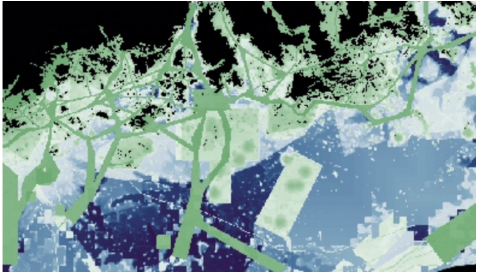
Mitä tummempi sininen väri, sen parempi tuulivoimapikka. Vihreä osoittaa laivaväylät, vaaleanvihreä suojeltavia alueita. Kuvakaappaus SYKEN tuulivoimatutkimuksen kartasta.
